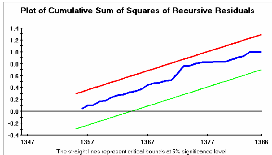
نمودار ۲. استحکام مدل با استفاده از آزمون CUSUM.SQ
