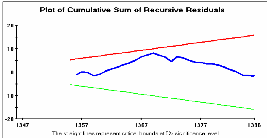
نمودار ۱. استحکام مدل با استفاده از آزمون CUSUM
