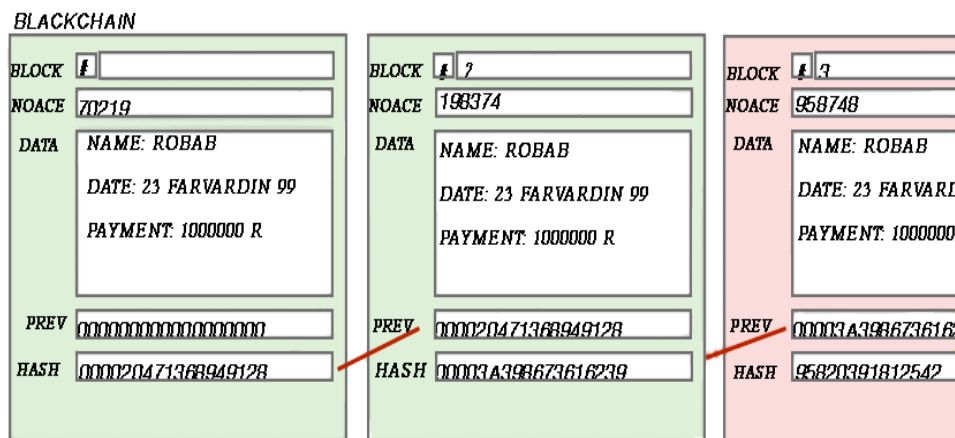
شکل ۱: عملکرد بلاکچین در بلوک‌های متوالی
